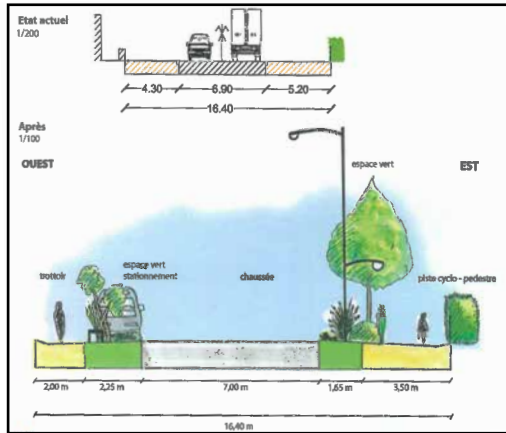
Coupe de principe - Zone Nord
