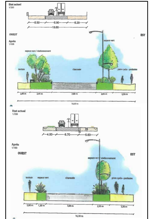
Coupes de principe - Zone Sud
