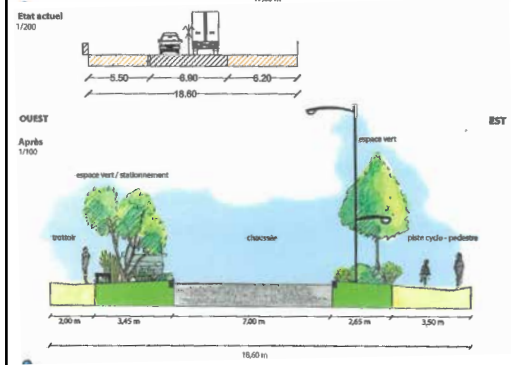
Coupes de principe - Zone centrale
