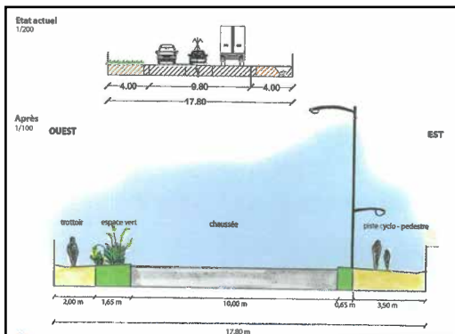
Coupe de principe - Zone Nord
